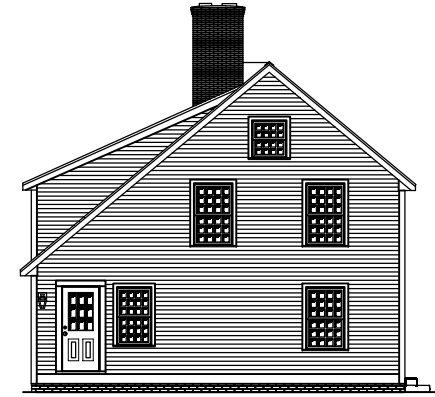
LEFT ELEVATION SCALE: 1/8" = 1'0"
